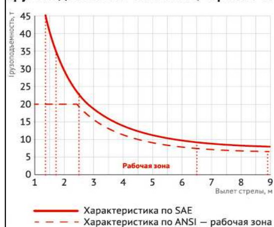
Грузоподъемность ТГ20.32Е2, стрела 9 м
