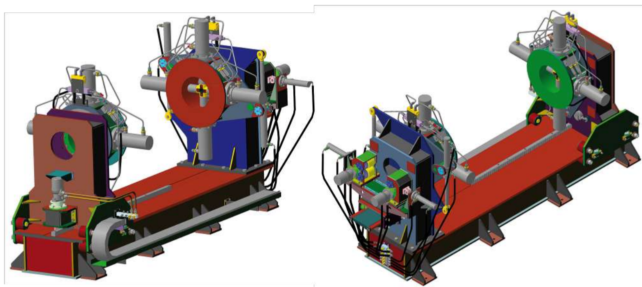
Ключ гидравлический стендовый для пакеров
